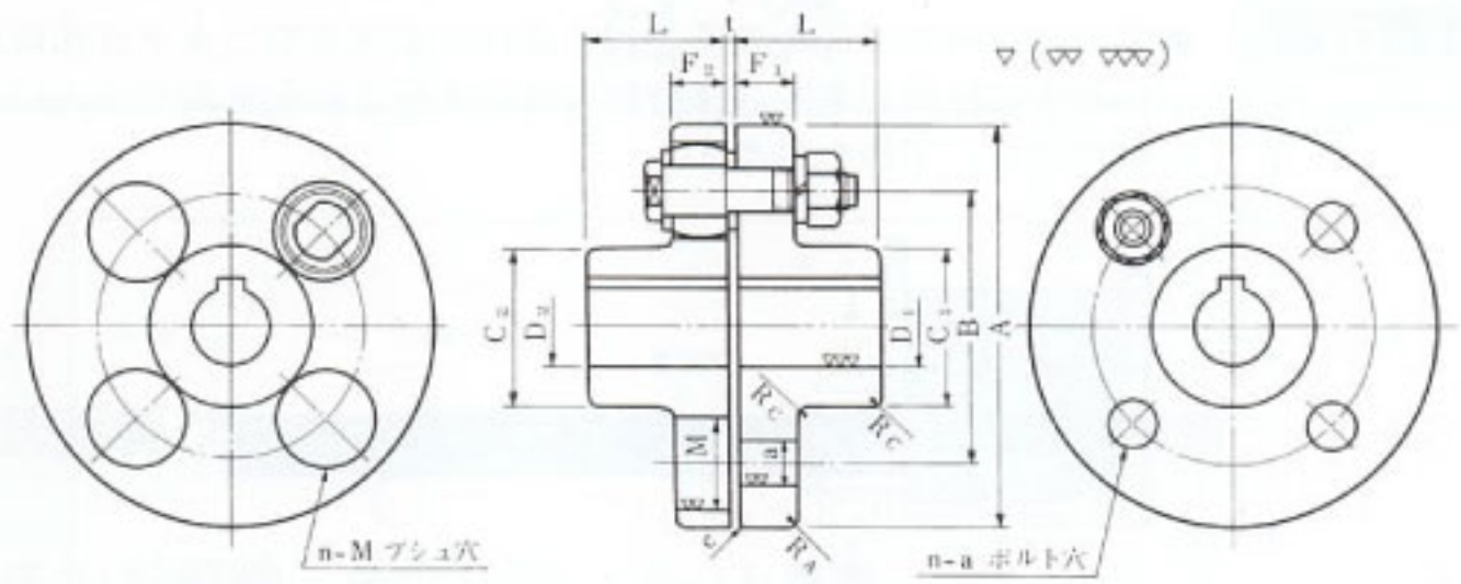
備考 ボルト穴の配置は、キー溝に対しておおむね振分けとする。
