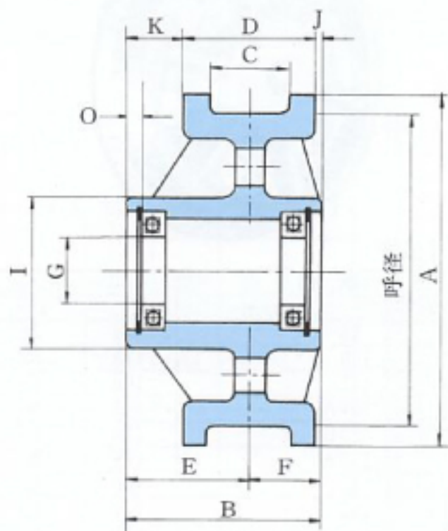
従動車
